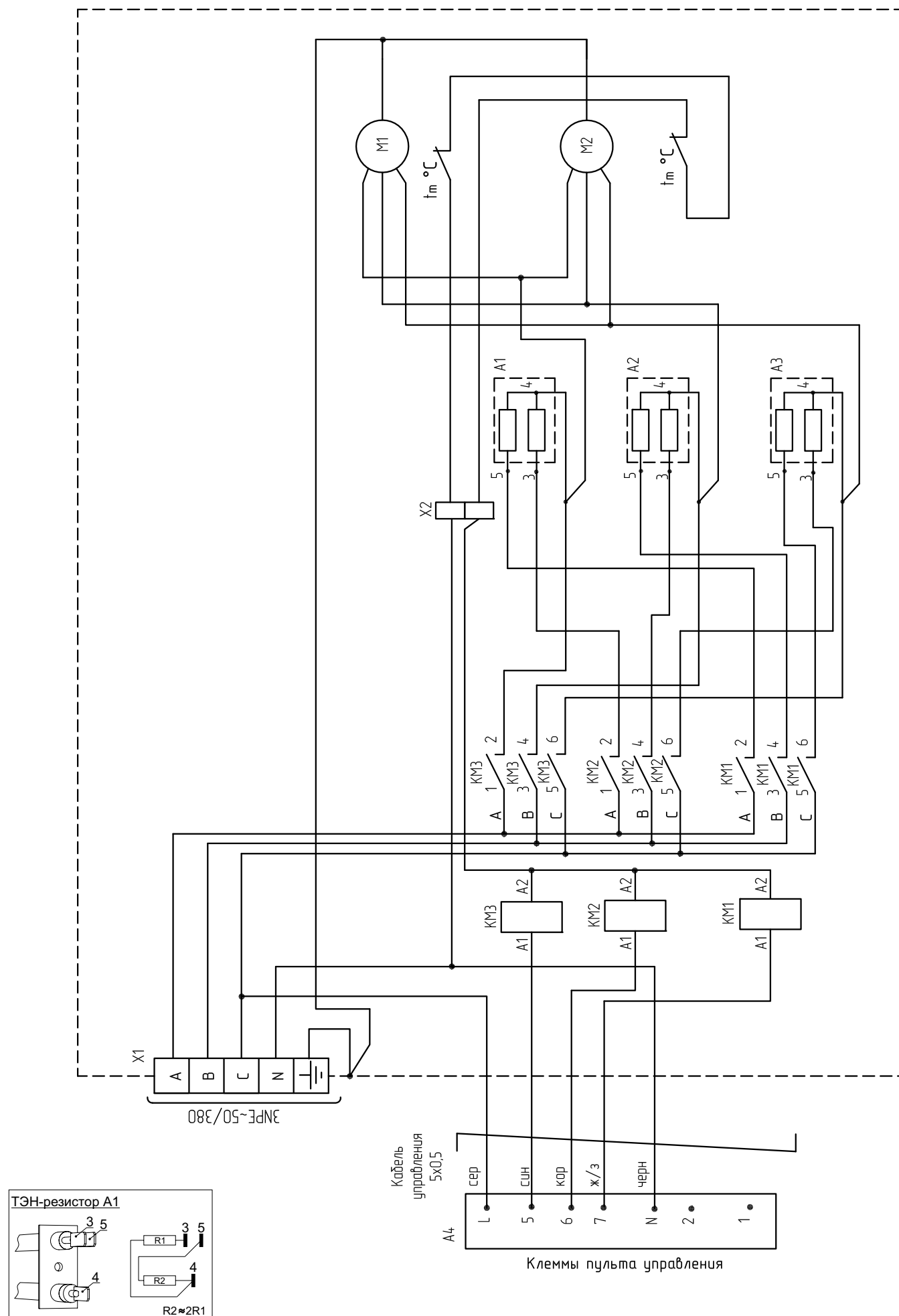
Рисунок 12. Электрическая схема занавесы КЭВ-170П7010W
